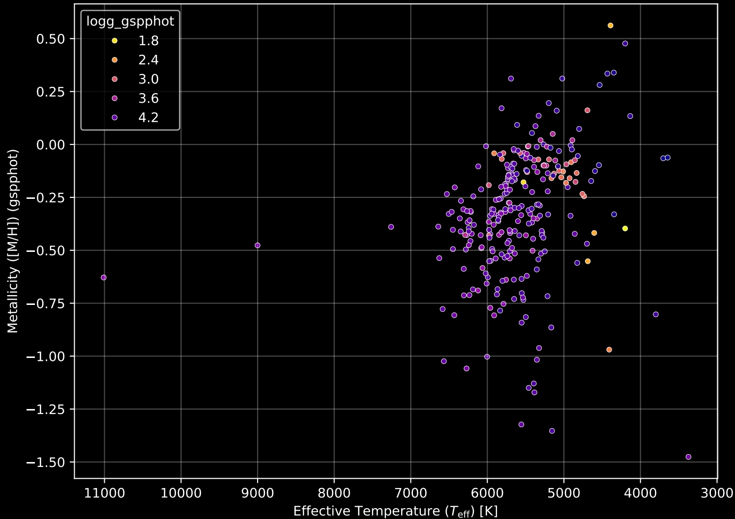
GALAH DR4 Field: [458] Stellar Population Parameters (n= 275)
