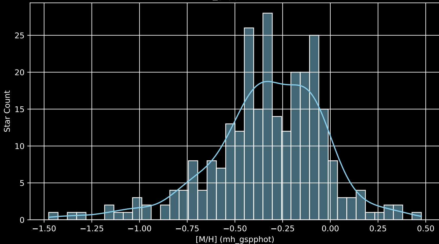
GALAH DR4 Field: [458] [M/H] (mh_gspphot) (n= 274)
