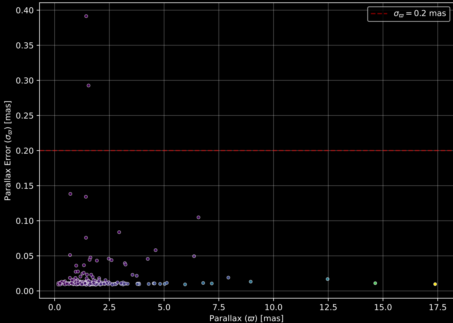
GALAH DR4 Field: [458] Parallax Quality (n= 275)
