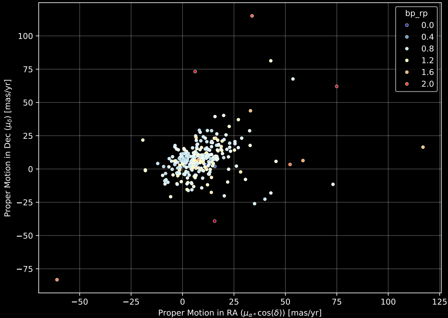
GALAH DR4 Field: [458] Proper Motion Diagram (n= 275)
